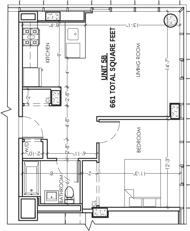
UNIT 5B SCALE: 1/8" = 1'-0"
