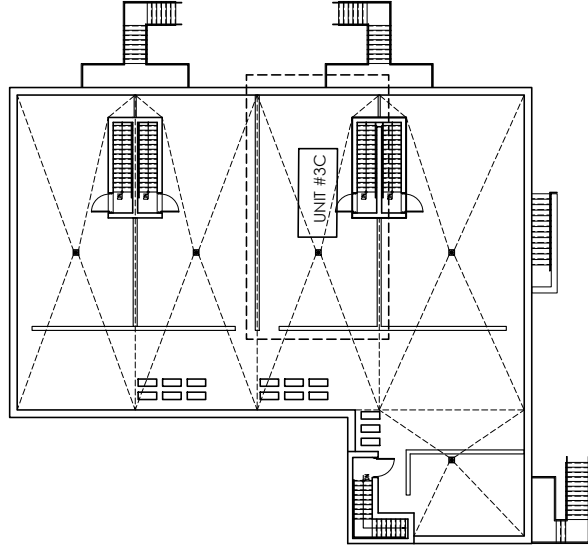
ROOF KEY PLAN N.T.S.
