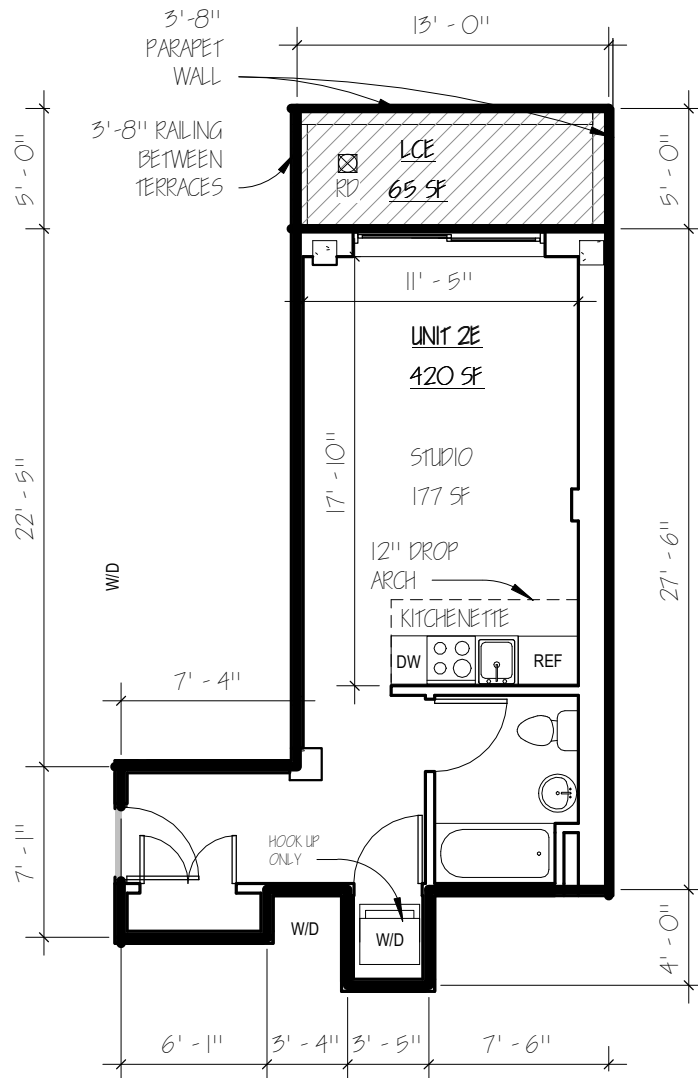
1 2 FL UNIT E 1/8" = 1'-0"
