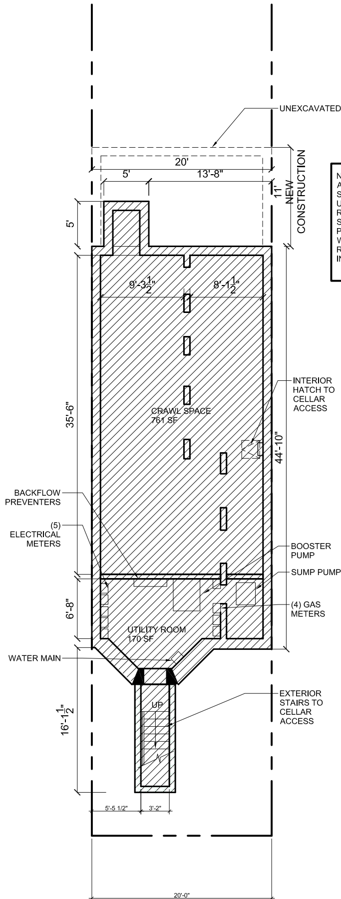
CELLAR FLOOR PLAN N.T.S.
