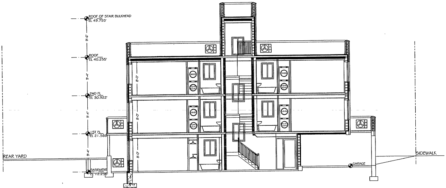
LONGITUDINAL SECTION
