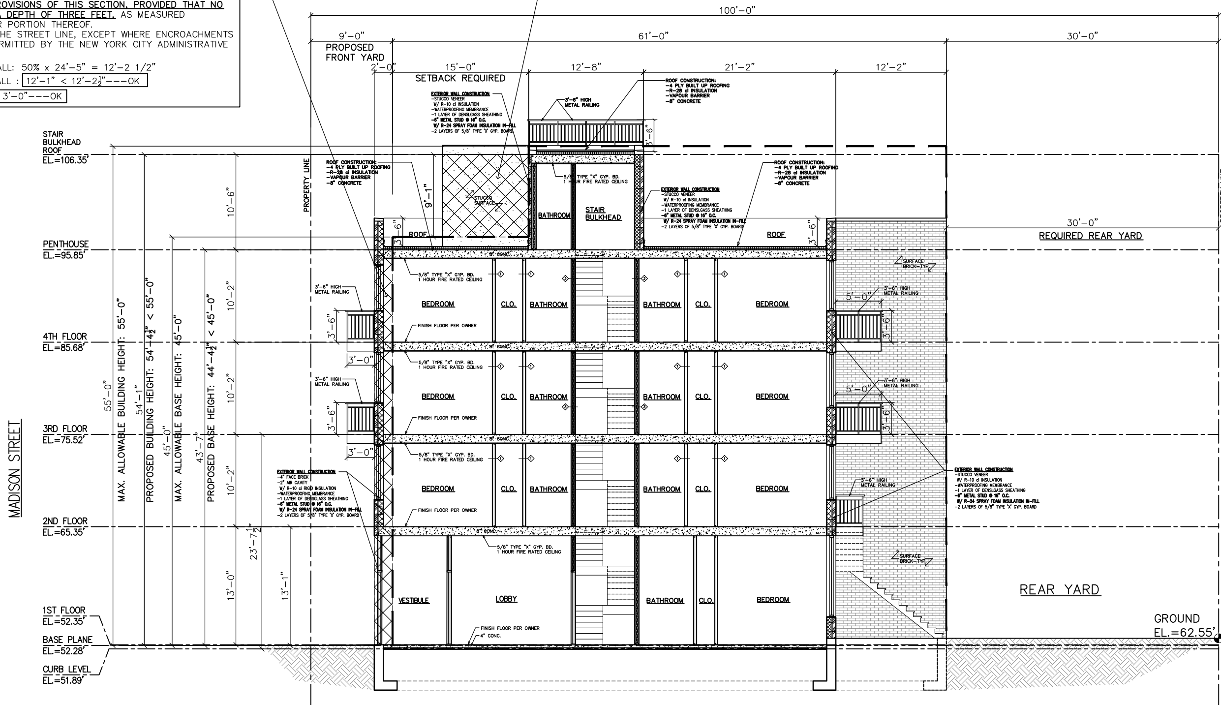
A BUILDING LONGITUDINAL SECTION A A04 SCALE: 3/16" = 1'-0"
