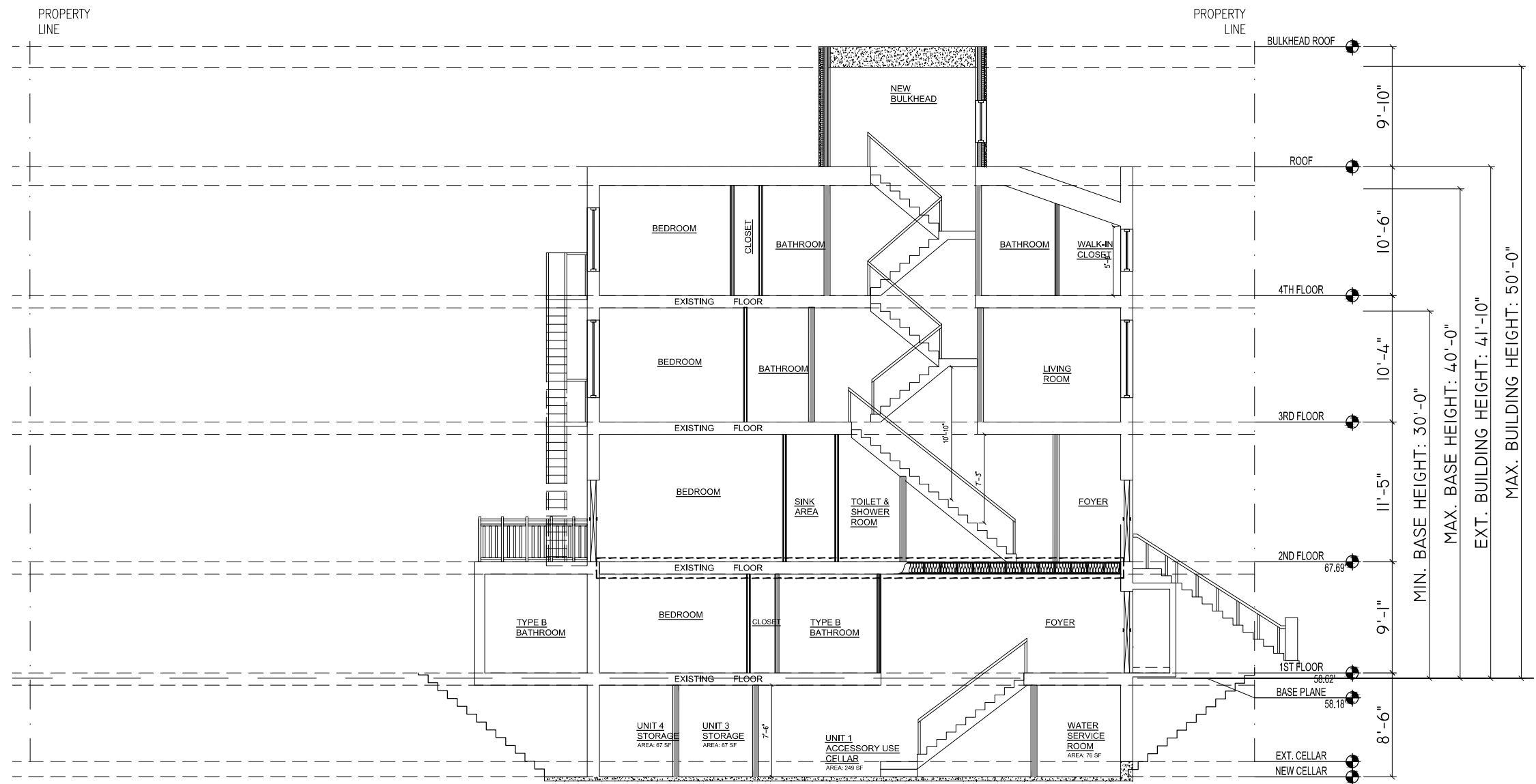
2 SECTION B SCALE: 1/4" = 1'-0"
