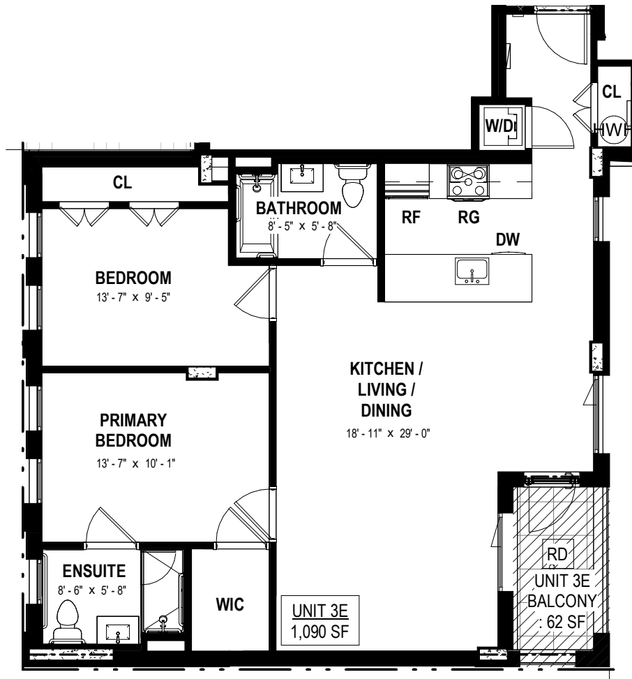
LEVEL 03 - UNIT 3E
