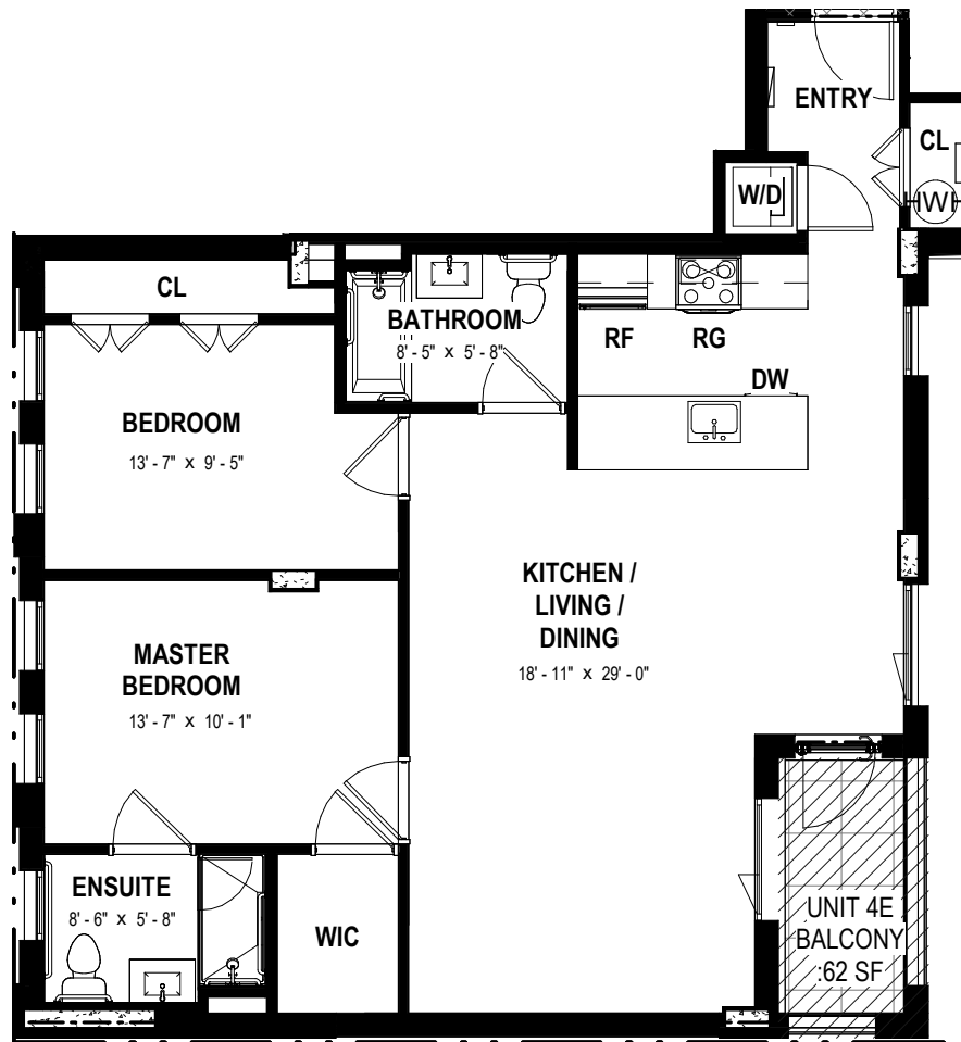
LEVEL 04 - UNIT 4E
