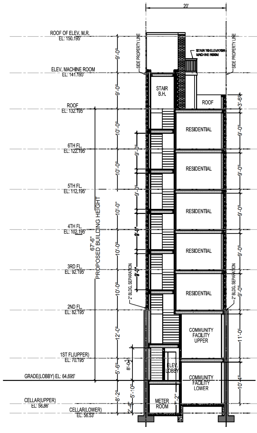
SECTION "B-B" N.T.S.
