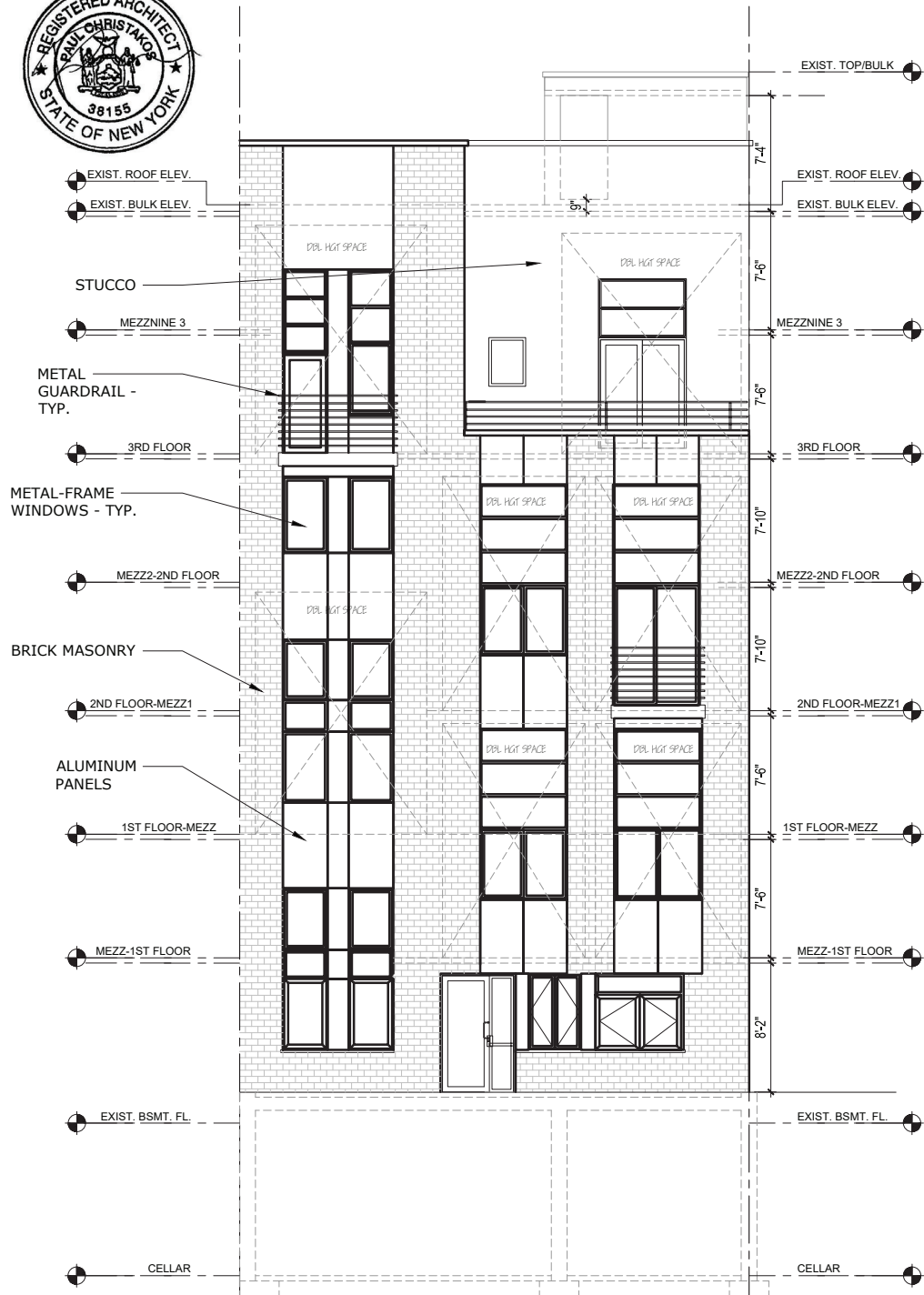
1 FRONT ELEVATION SCALE: 1/8" = 1'-0"
